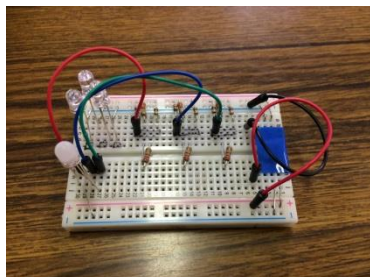
図1 抵抗による光の制御
