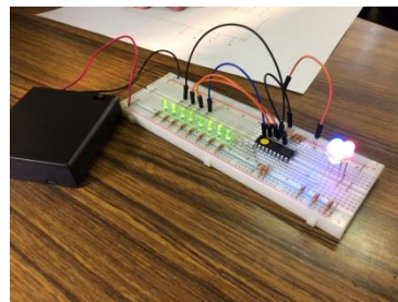
図2 時間による光の制御
